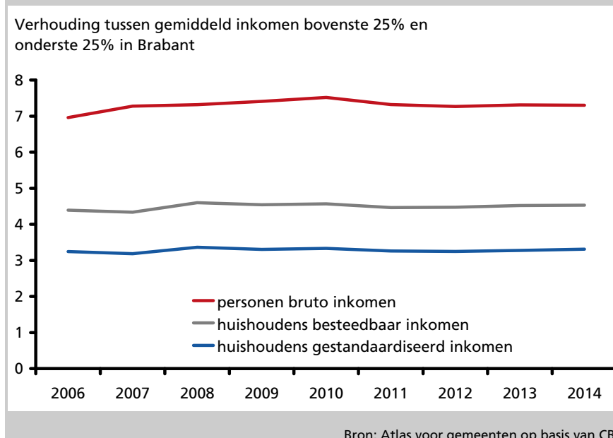
Figuur 4.5 De inkomensongelijkheid in Brabant is vrijwel constant
