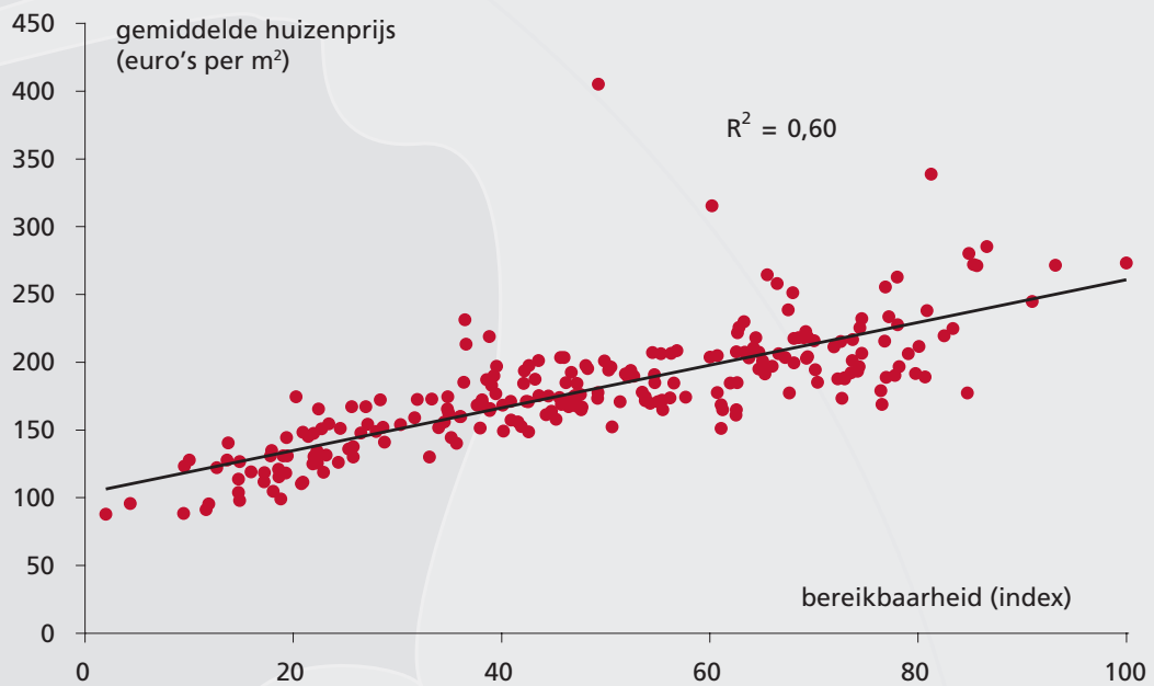
Figuur 4 Verschillen in huizenprijzen verklaard door bereikbaarheid, per auto en OV, alle Nederlandse gemeenten
